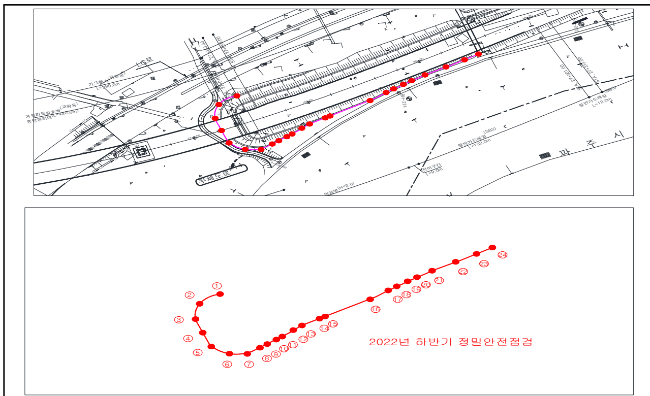
【그림 8.11】 계획선형 측량 현황
